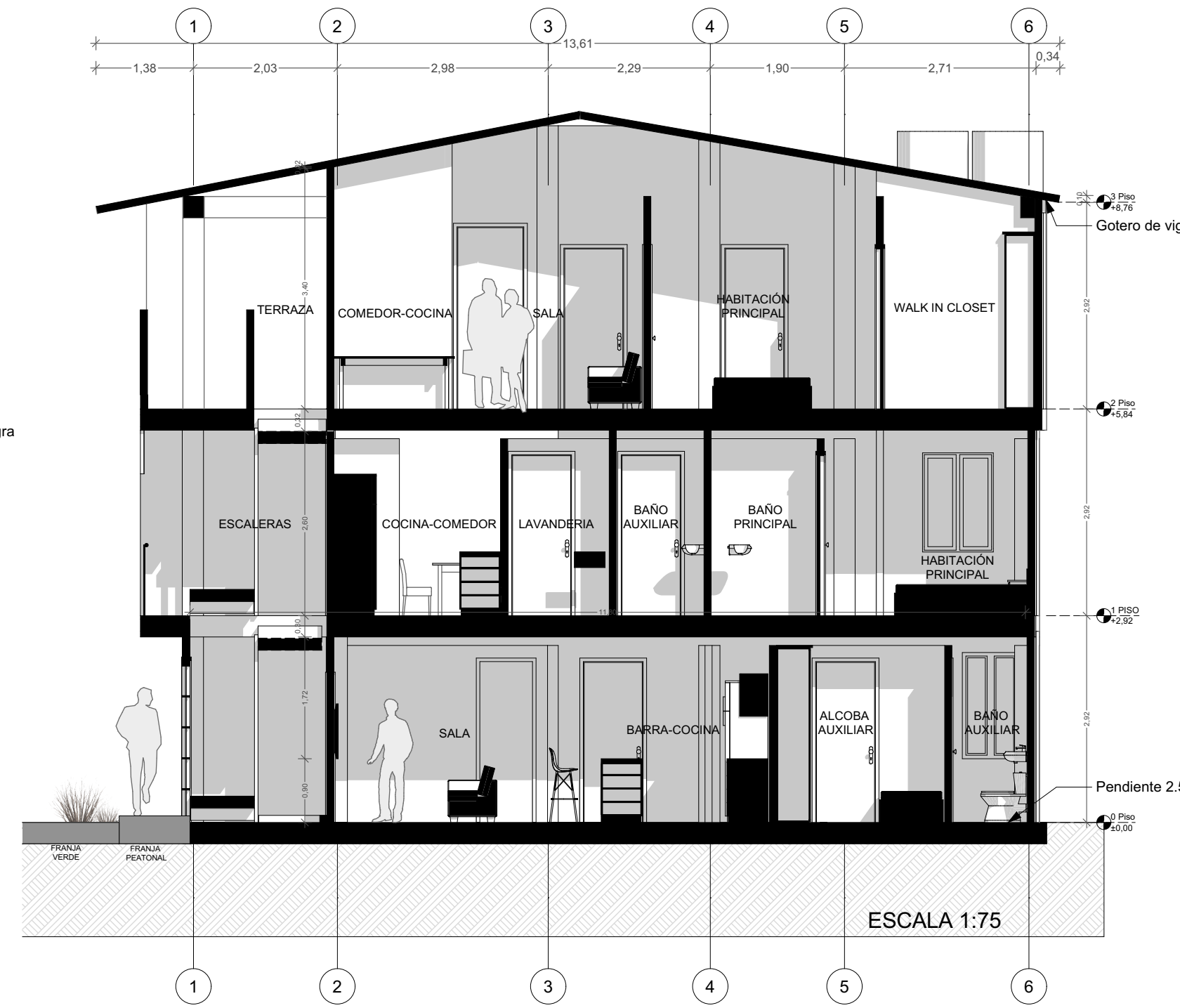
CORTE LONGITUDINAL
