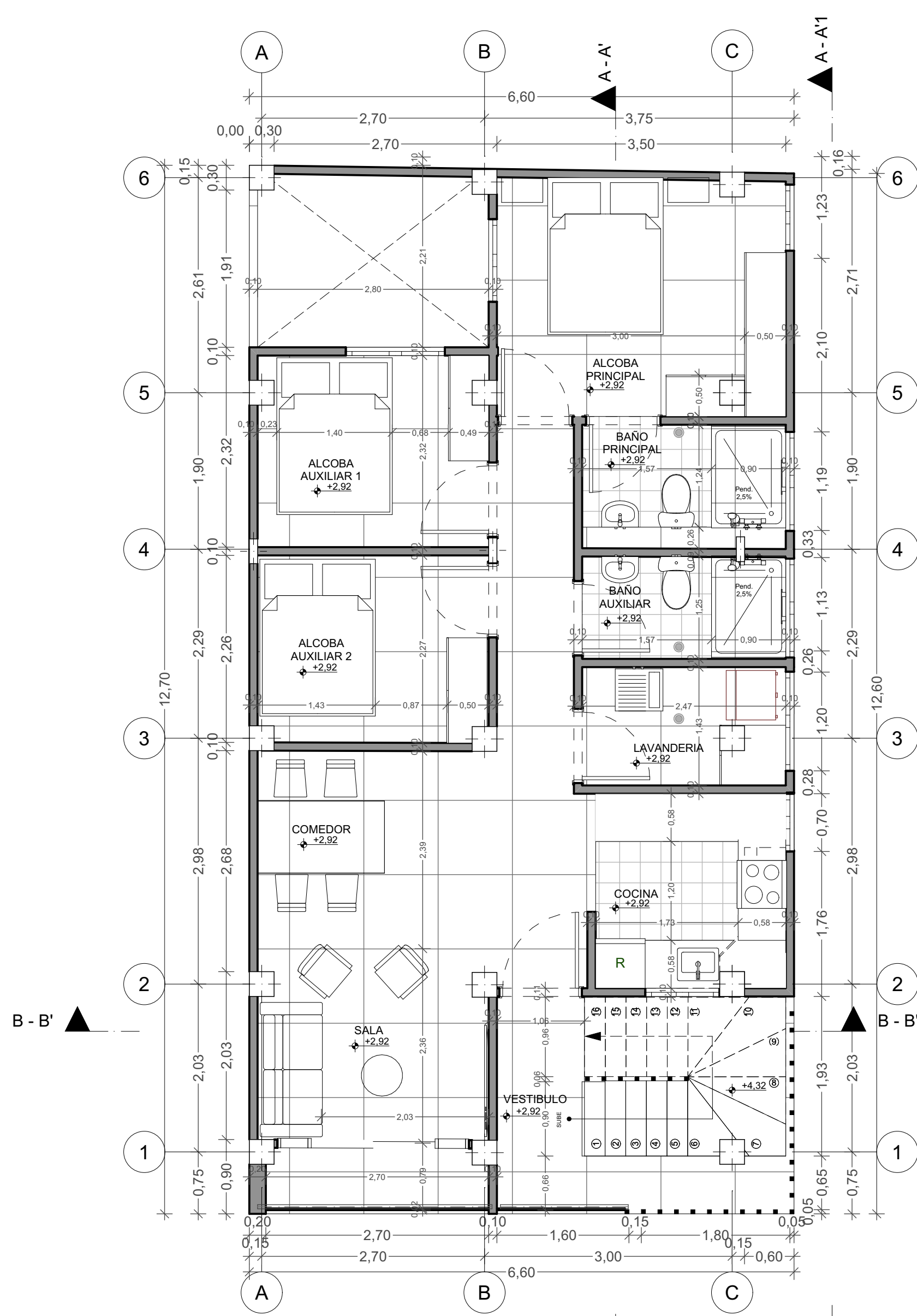
PLANTA SEGUNDO PISO
