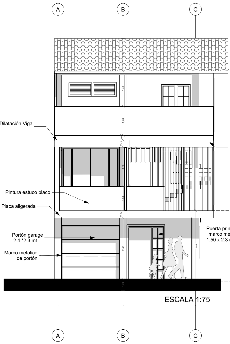
FACHADA FRONTAL
