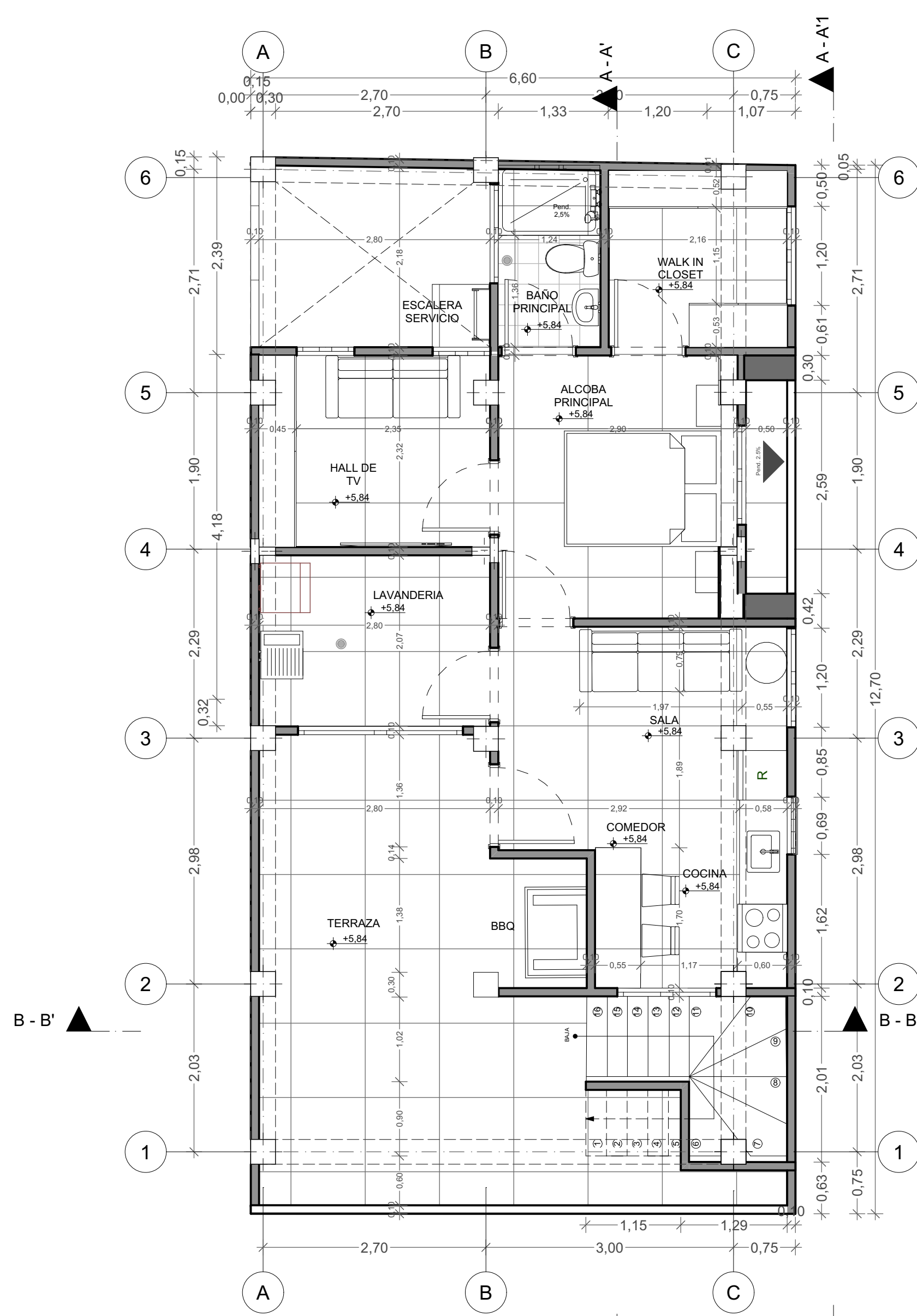
PLANTA TERCER PISO
