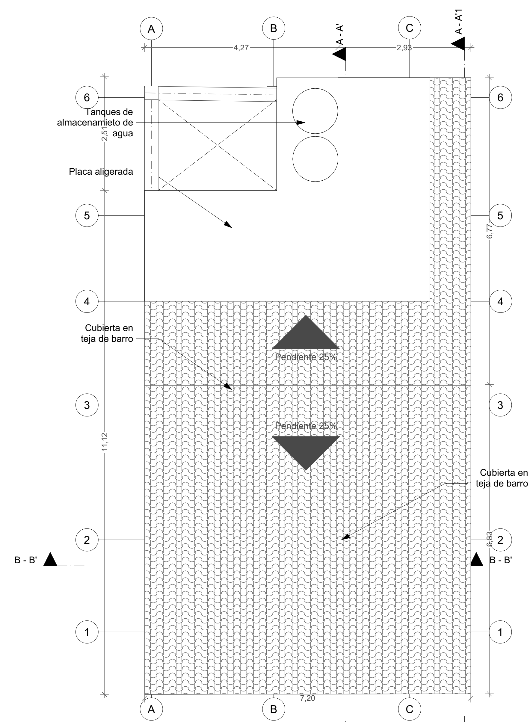
PLANTA DE CUBIERTA
