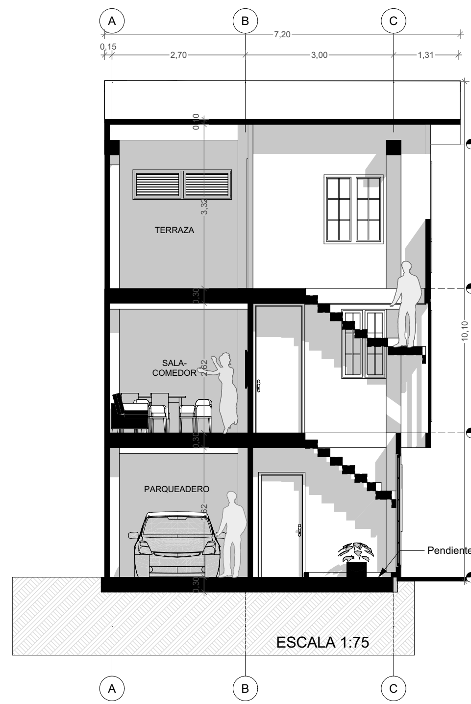
CORTE TRANSVERSAL
